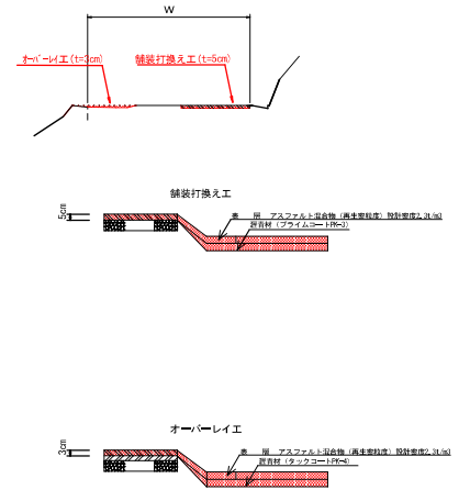
標準断面図 S=1/100
